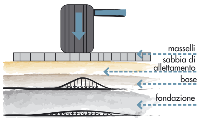
fig. 4.2 - Tensioni critiche in una sovrastruttura di tipo flessibile
